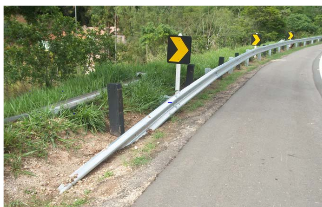
Figura 4 – Ancoragem de Defesa
