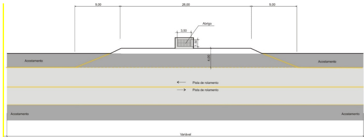
Figura 12– Projeto Padrão para Baia de Parada de Ônibus com Abrigo de Passageiros
