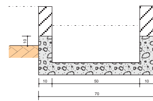
CORTE TRANSVERSAL B B'
