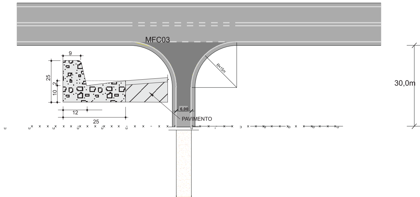
SEÇÃO TRANSVERSAL TIPO - ACESSOS SECUNDÁRIOS
