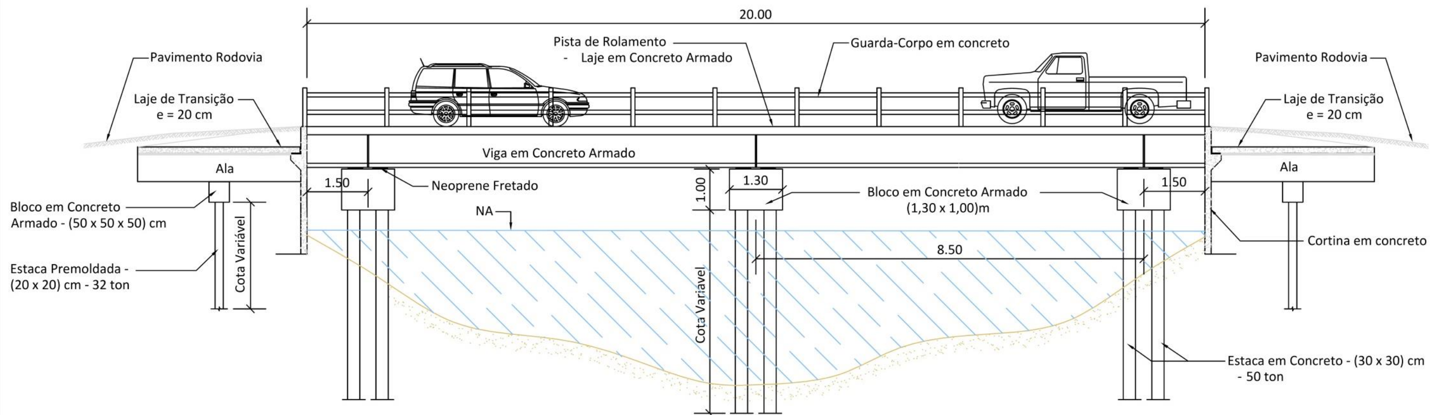
SEÇÃO 01 - LONGITUDINAL
