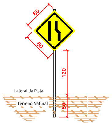
PLACA DE ESTREITAMENTO DE PISTA À DIREITA
