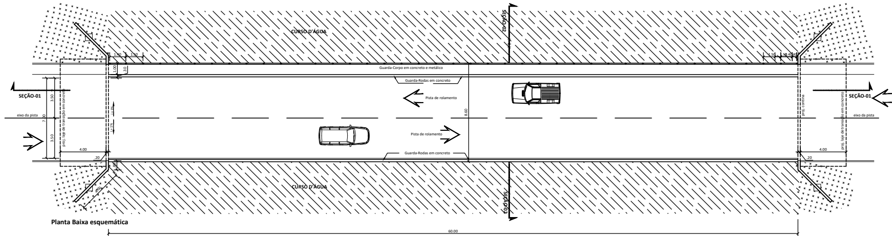
DETALHE 01 - LAJE DE TRANSIÇÃO E PISTA DE ROLAMENTO
