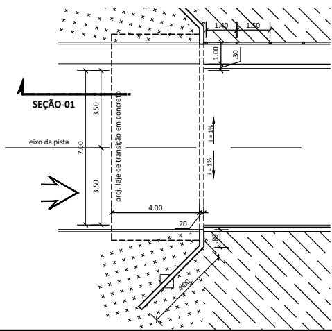
DETALHE 01 - LAJE DE TRANSIÇÃO E PISTA DE ROLAMENTO
