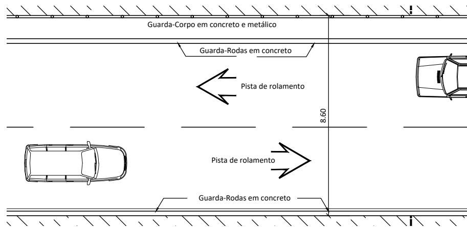
DETALHE 02 - PISTA DE ROLAMENTO E PASSARELA
