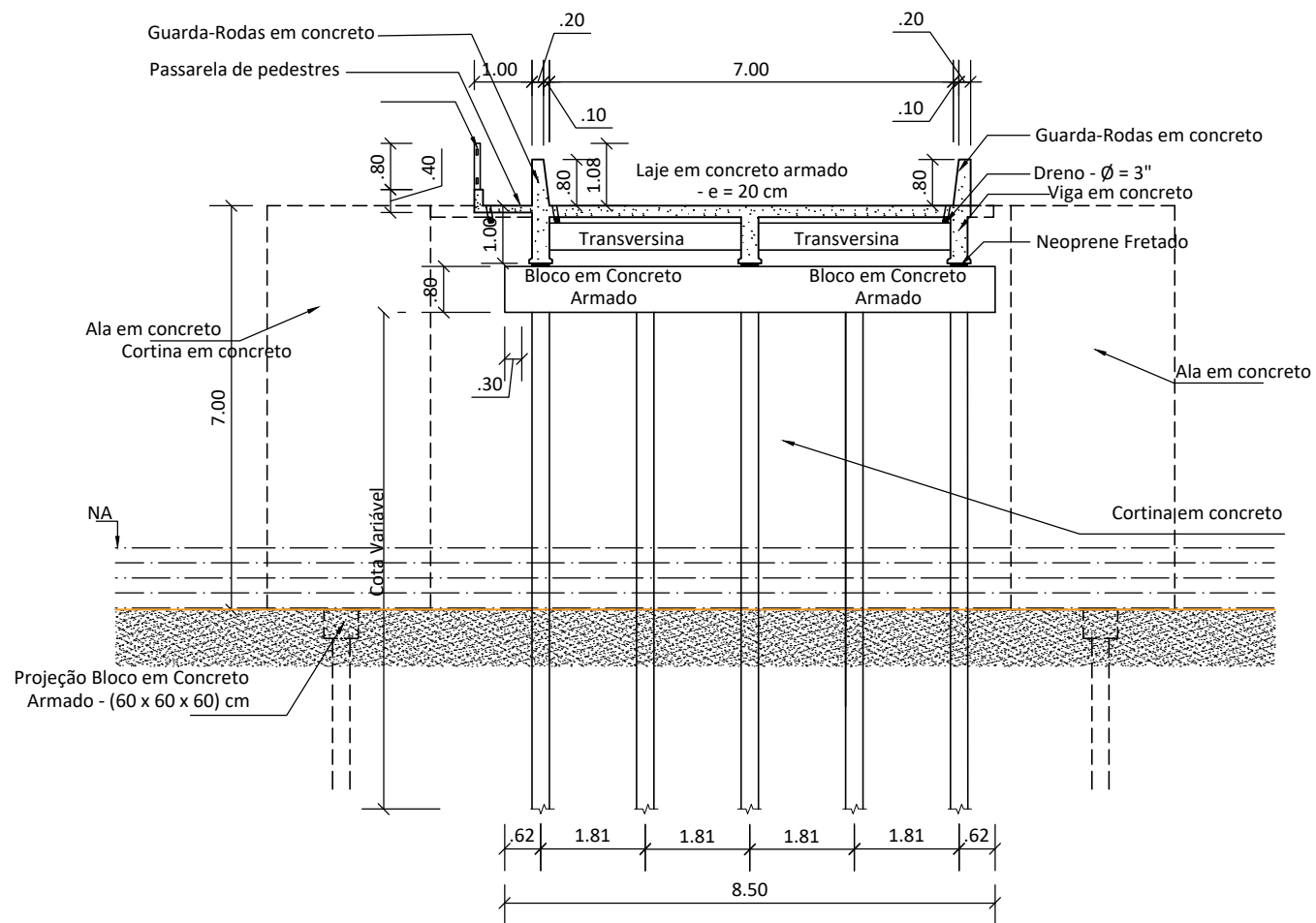
SEÇÃO 02 - TRANSVERSAL
