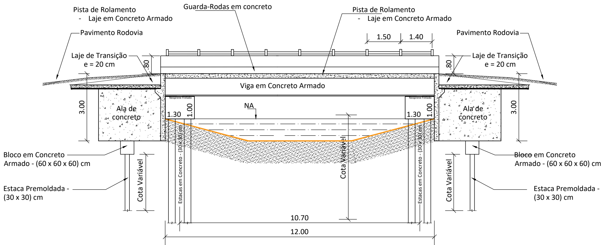
SEÇÃO 01 - LONGITUDINAL
