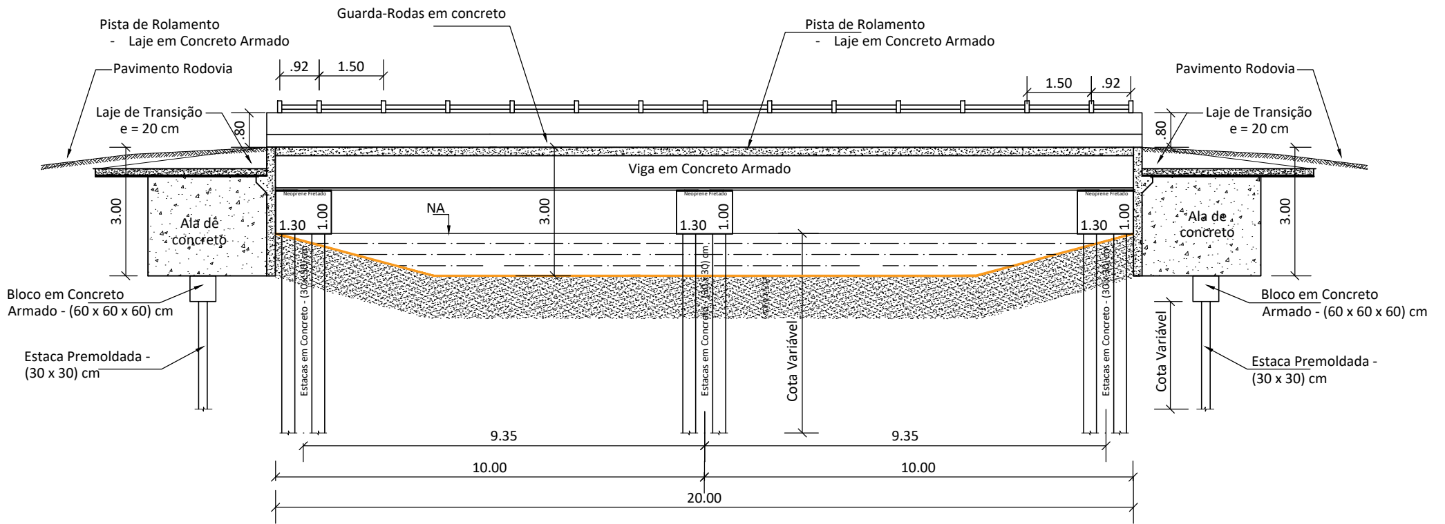
SEÇÃO 01 - LONGITUDINAL
