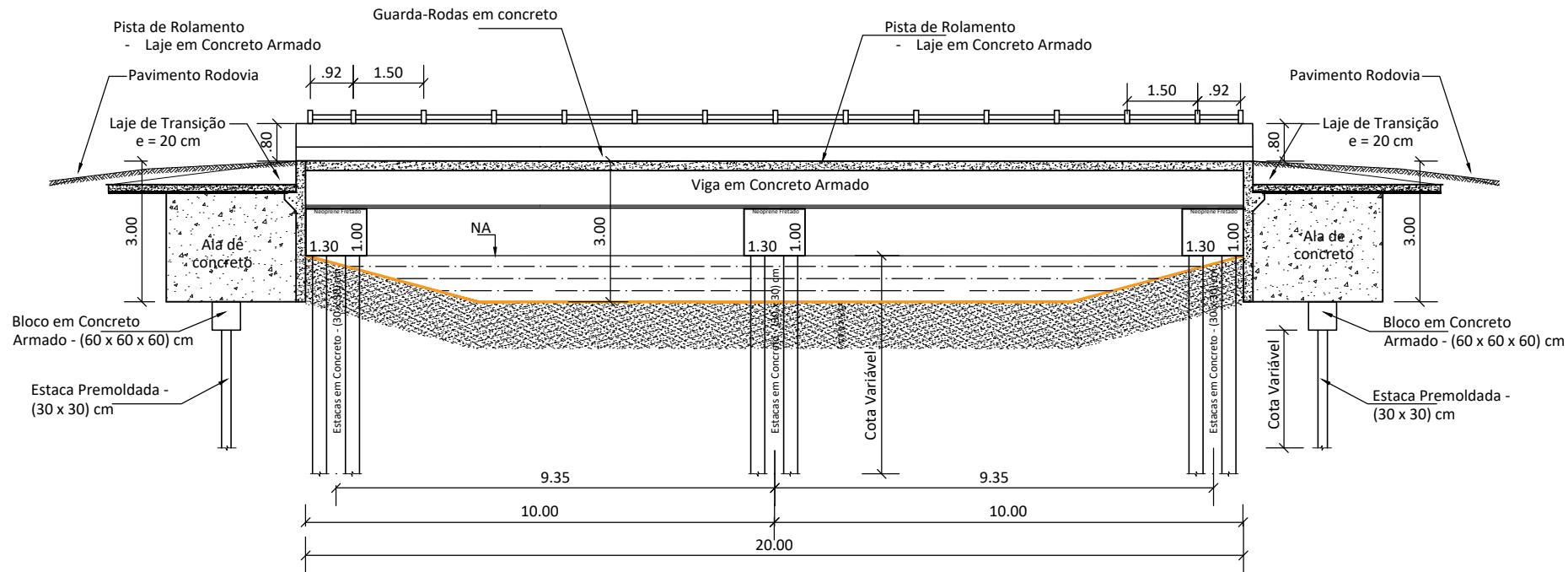
SEÇÃO 01 - LONGITUDINAL
