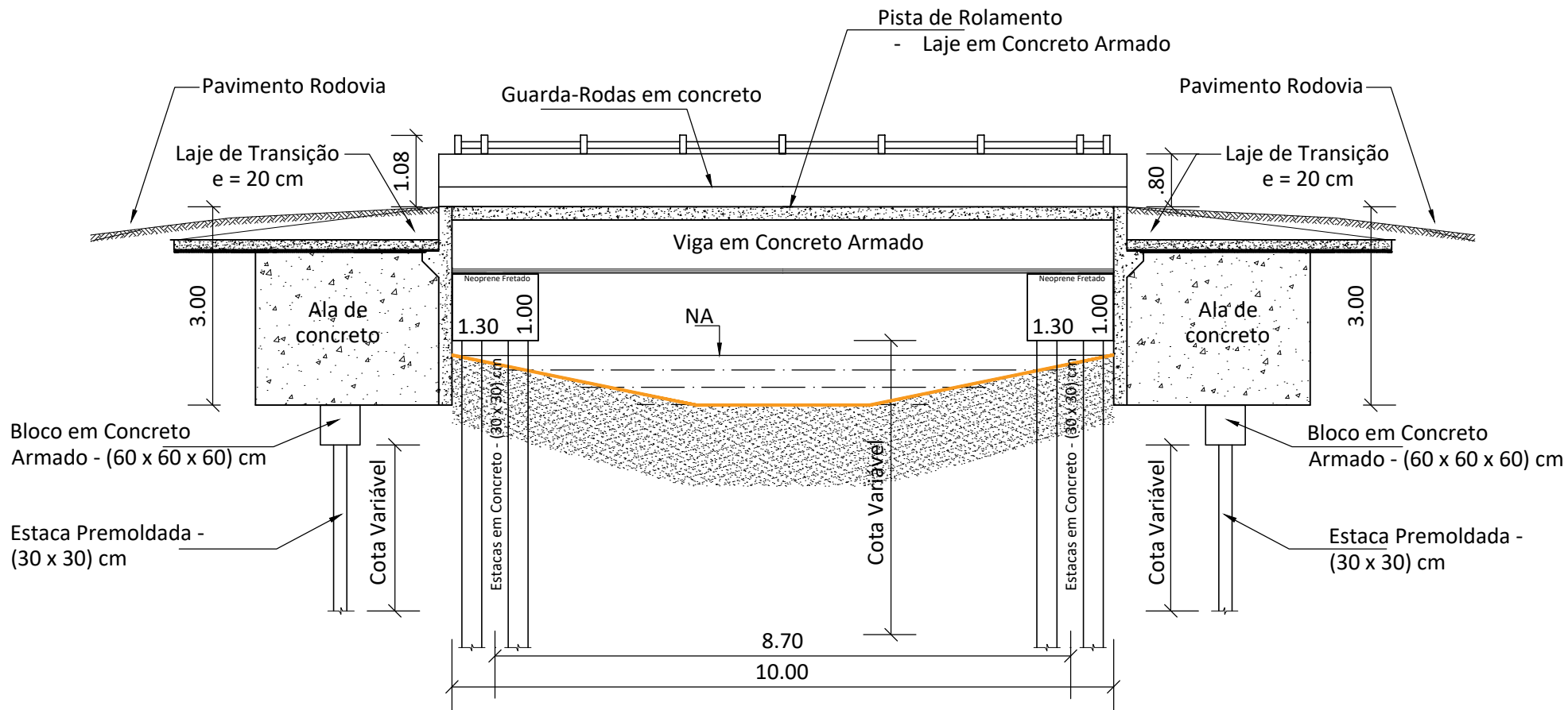
SEÇÃO 01 - LONGITUDINAL
