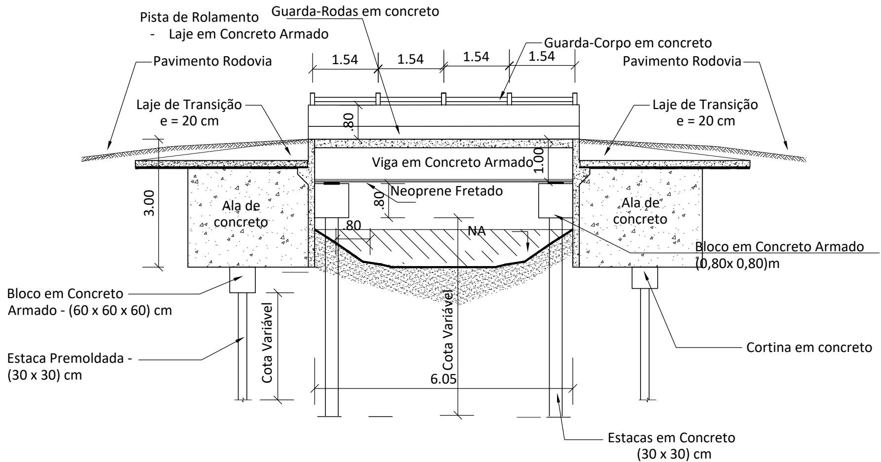
SEÇÃO 01 - LONGITUDINAL
