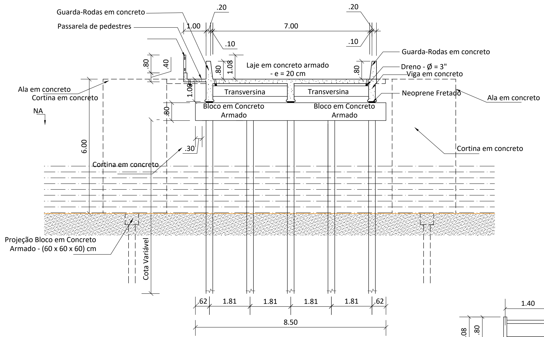
SEÇÃO 02 - TRANSVERSAL
