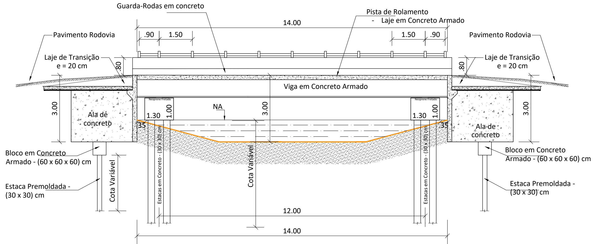
SEÇÃO 01 - LONGITUDINAL
