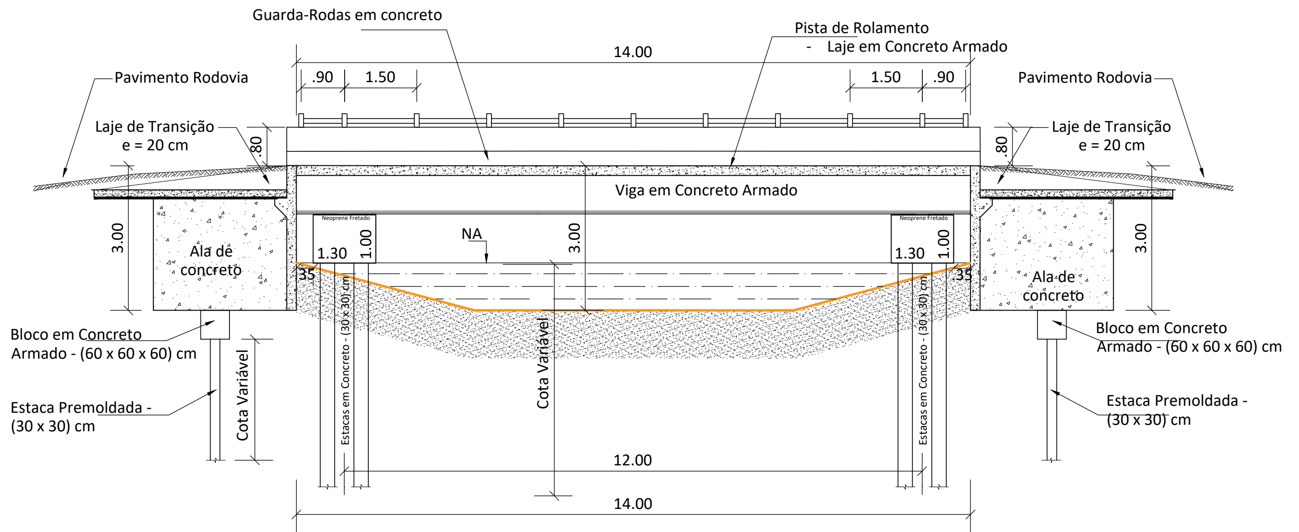
SEÇÃO 01 - LONGITUDINAL
