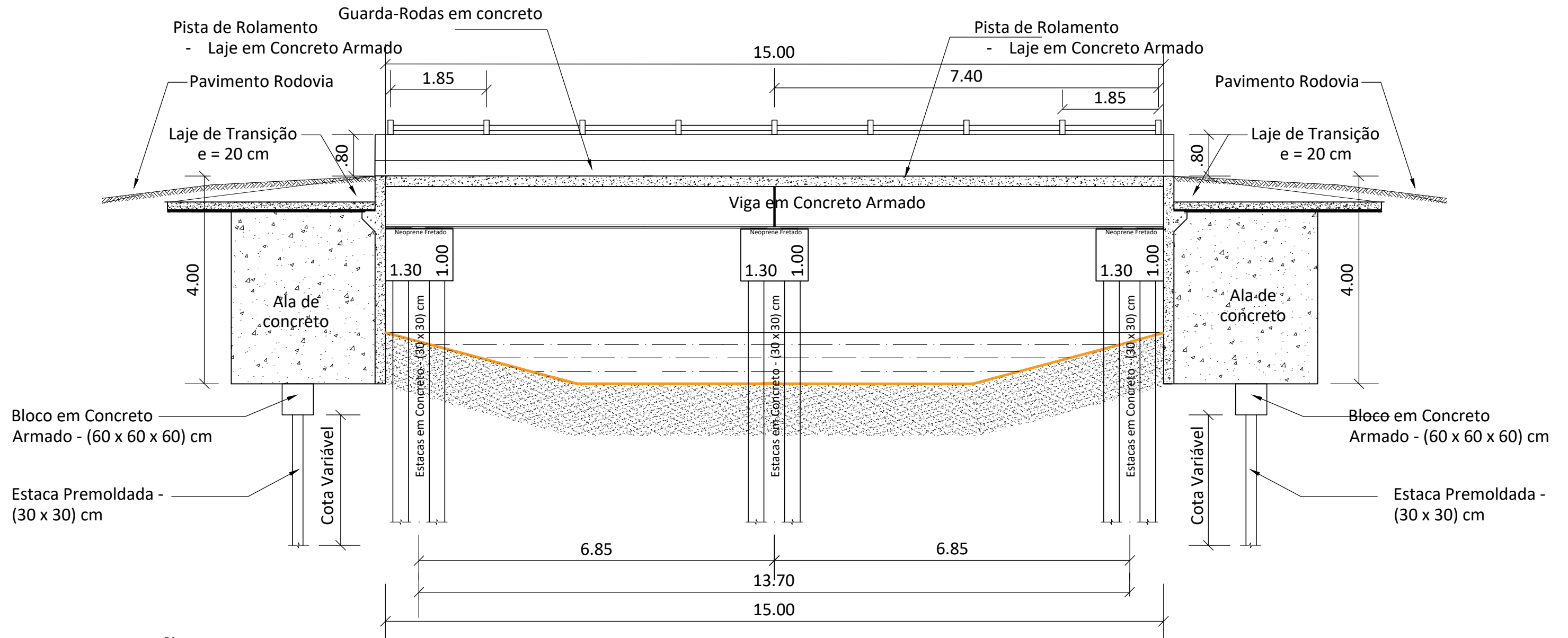
SEÇÃO 01 - LONGITUDINAL - ESCALA: 1 / 125
