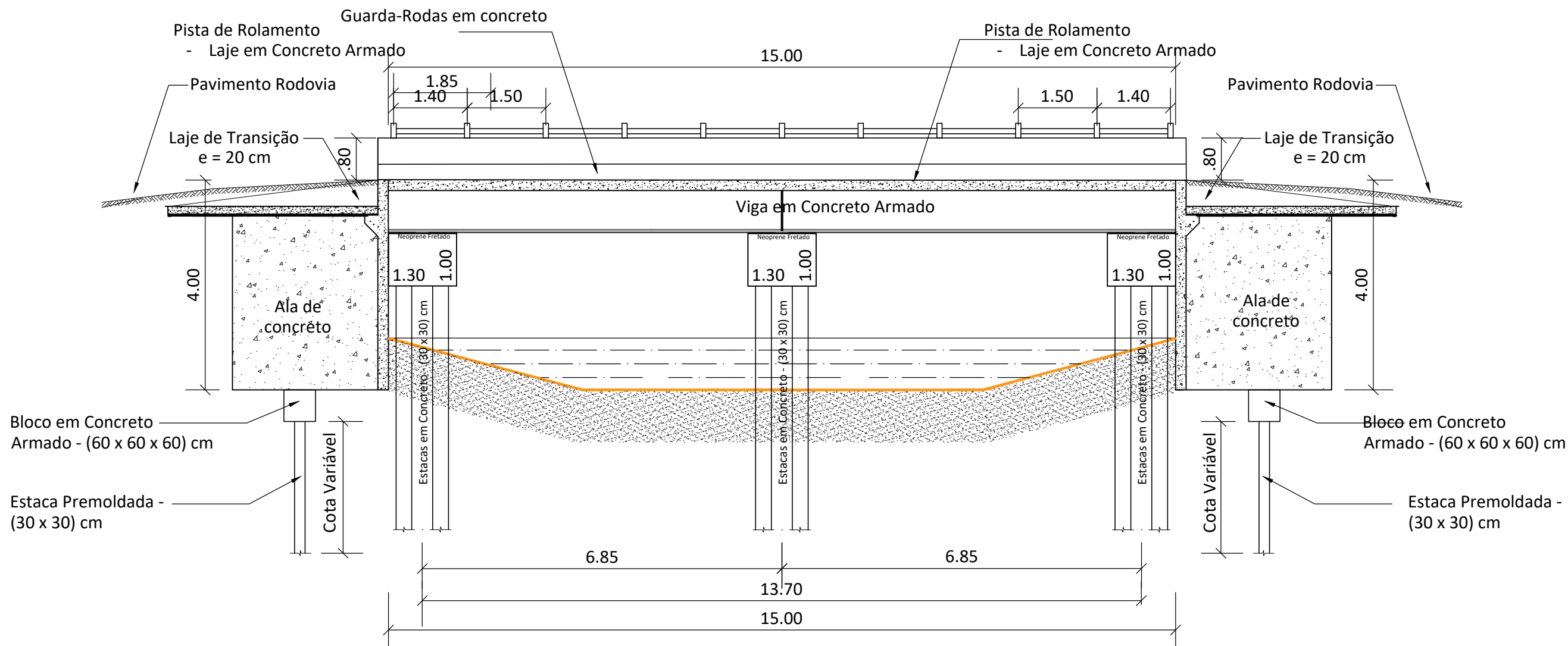
SEÇÃO 01 - LONGITUDINAL - ESCALA: 1 / 125
