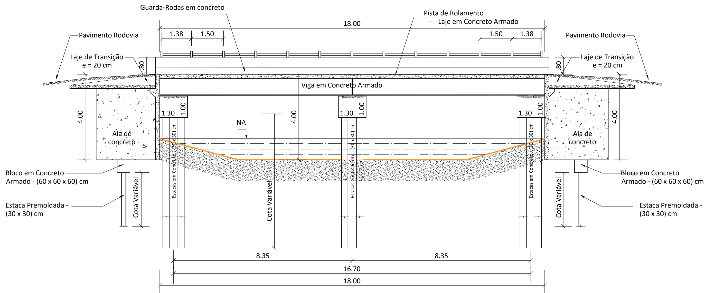
SEÇÃO 01 - LONGITUDINAL
