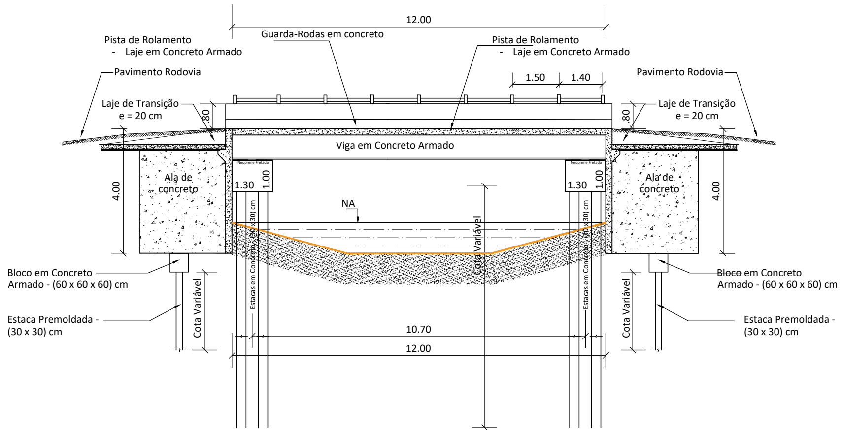
SEÇÃO 01 - LONGITUDINAL
