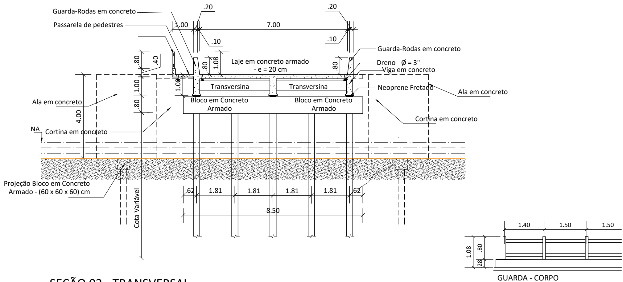
SEÇÃO 02 - TRANSVERSAL
