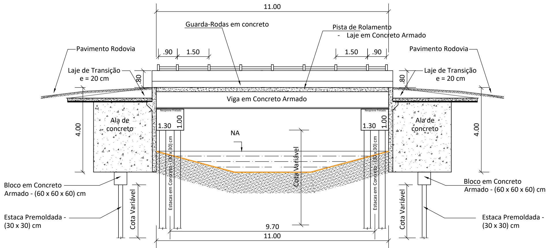
SEÇÃO 01 - LONGITUDINAL
