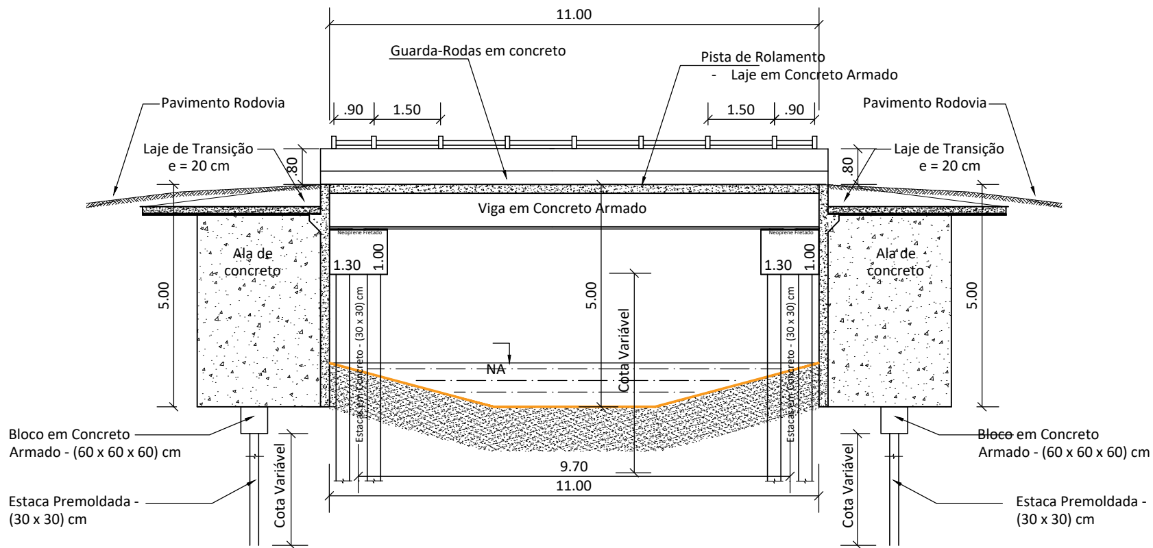
SEÇÃO 01 - LONGITUDINAL
