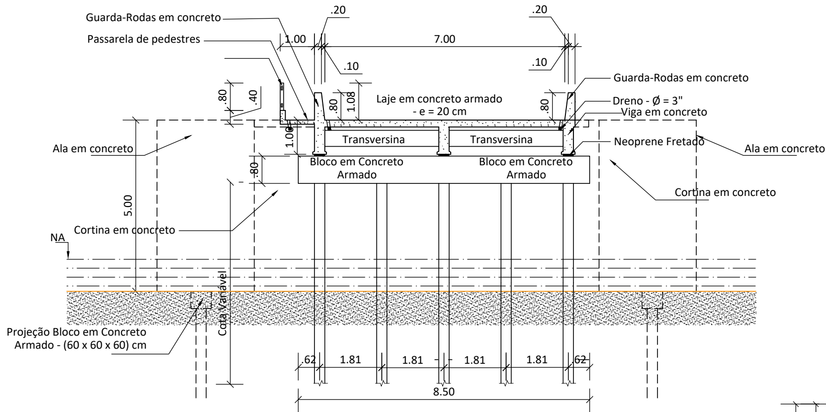
SEÇÃO 02 - TRANSVERSAL
