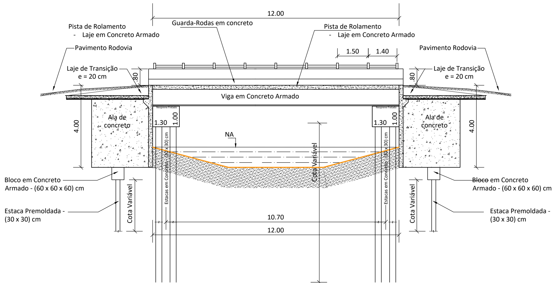
SEÇÃO 01 - LONGITUDINAL
