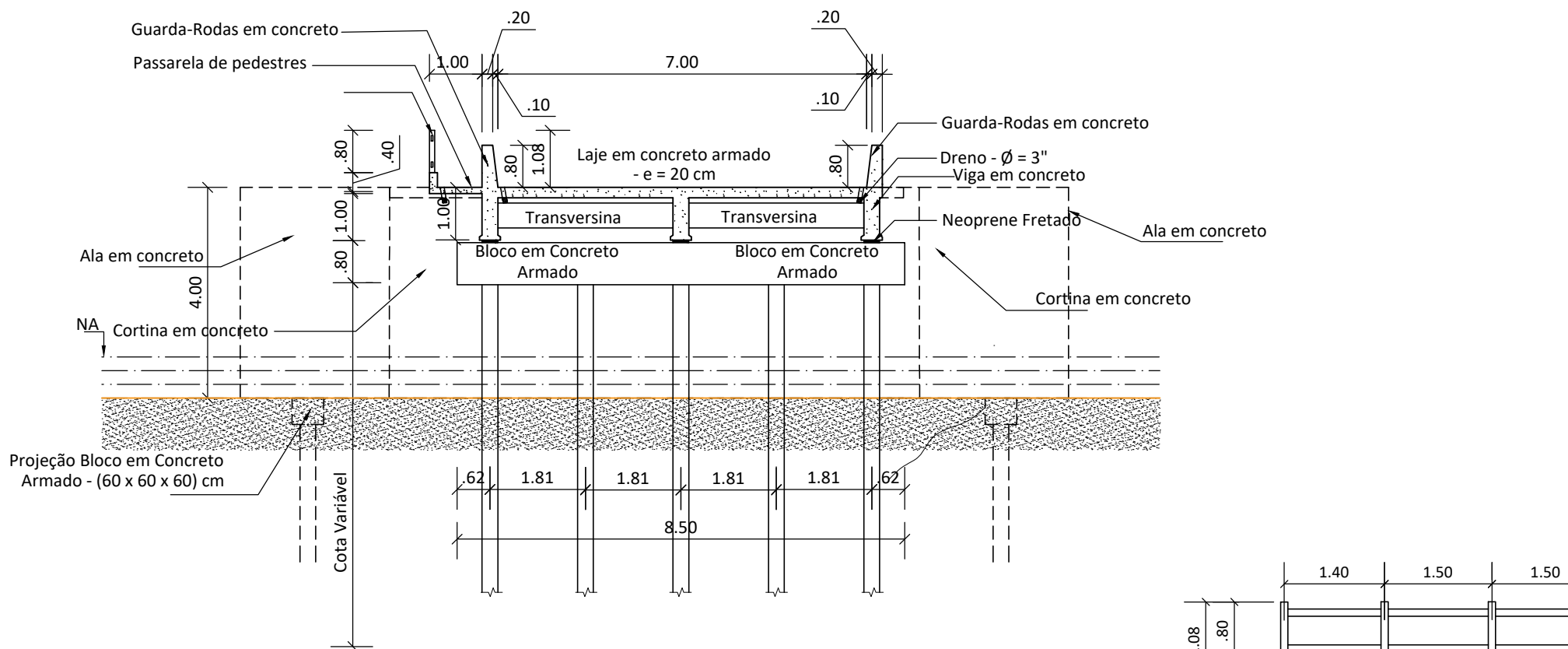
SEÇÃO 02 - TRANSVERSAL
