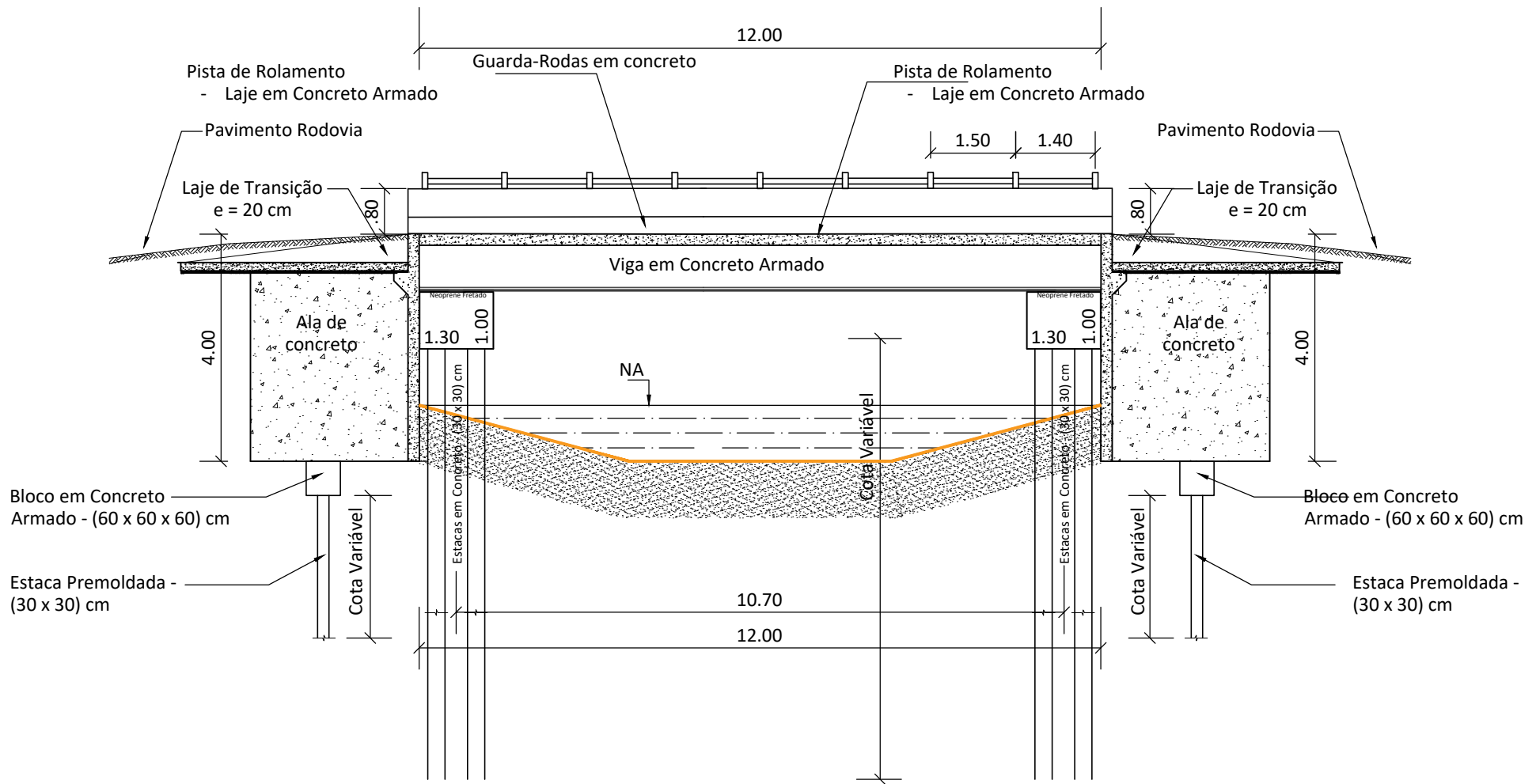
SEÇÃO 01 - LONGITUDINAL
