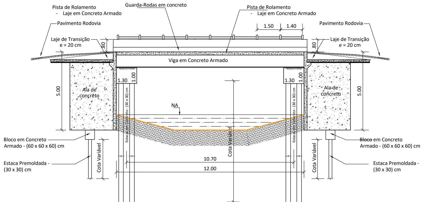
SEÇÃO 01 - LONGITUDINAL
