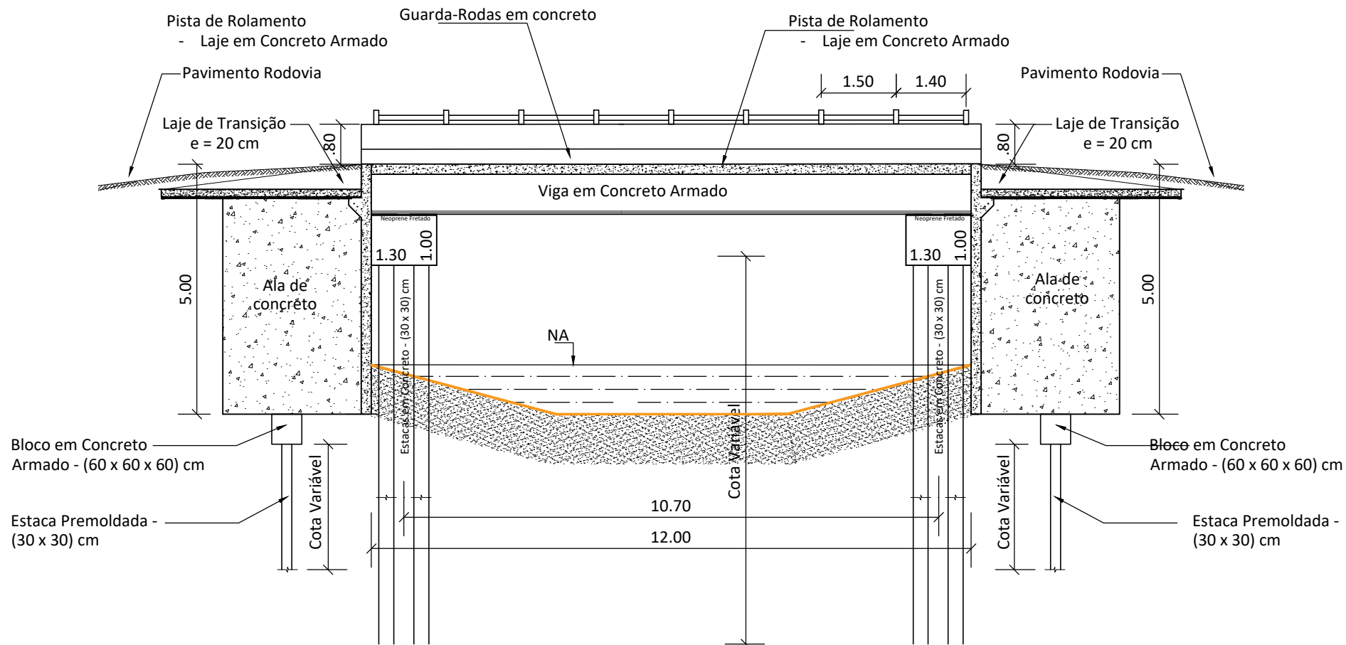
SEÇÃO 01 - LONGITUDINAL
