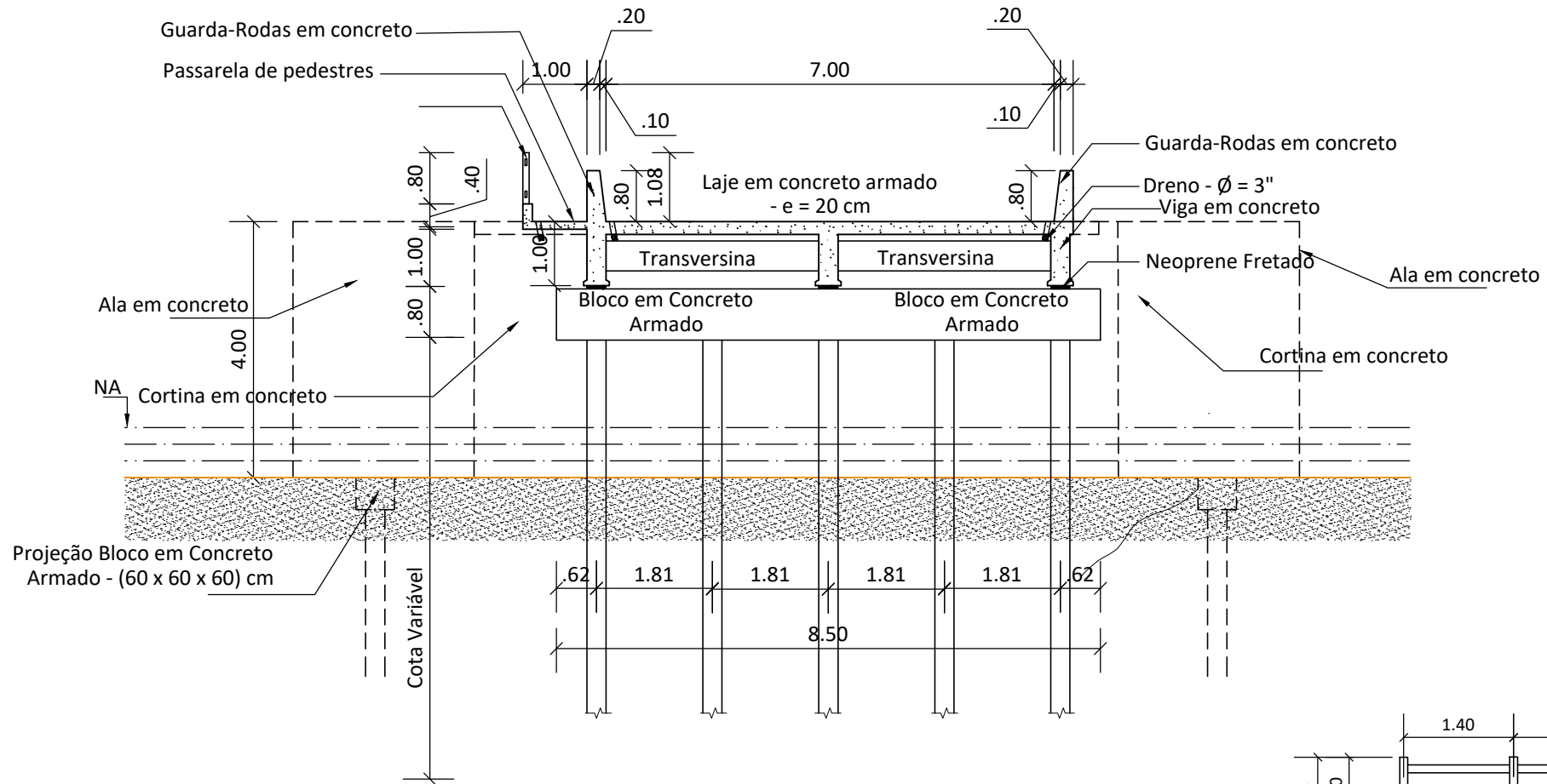
SEÇÃO 02 - TRANSVERSAL
