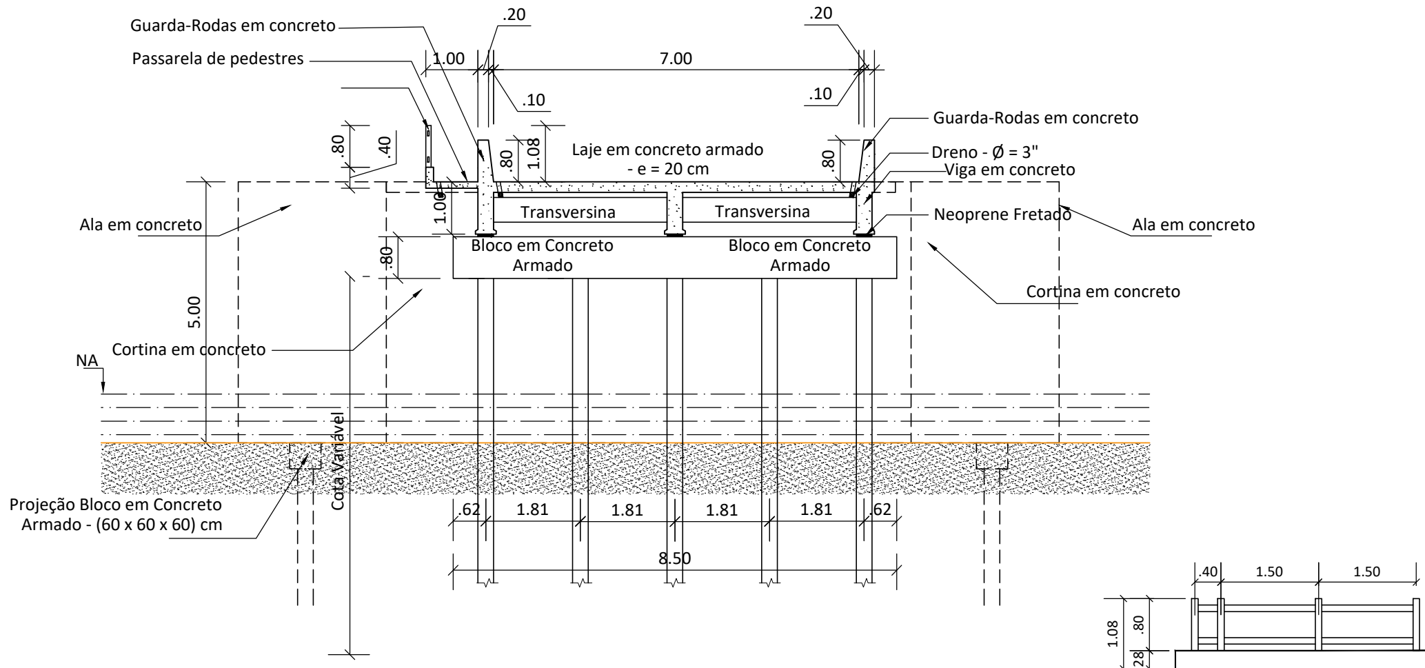
SEÇÃO 02 - TRANSVERSAL
