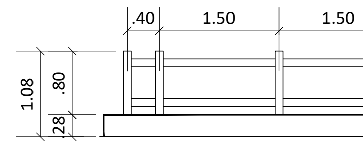
GUARDA - CORPO
