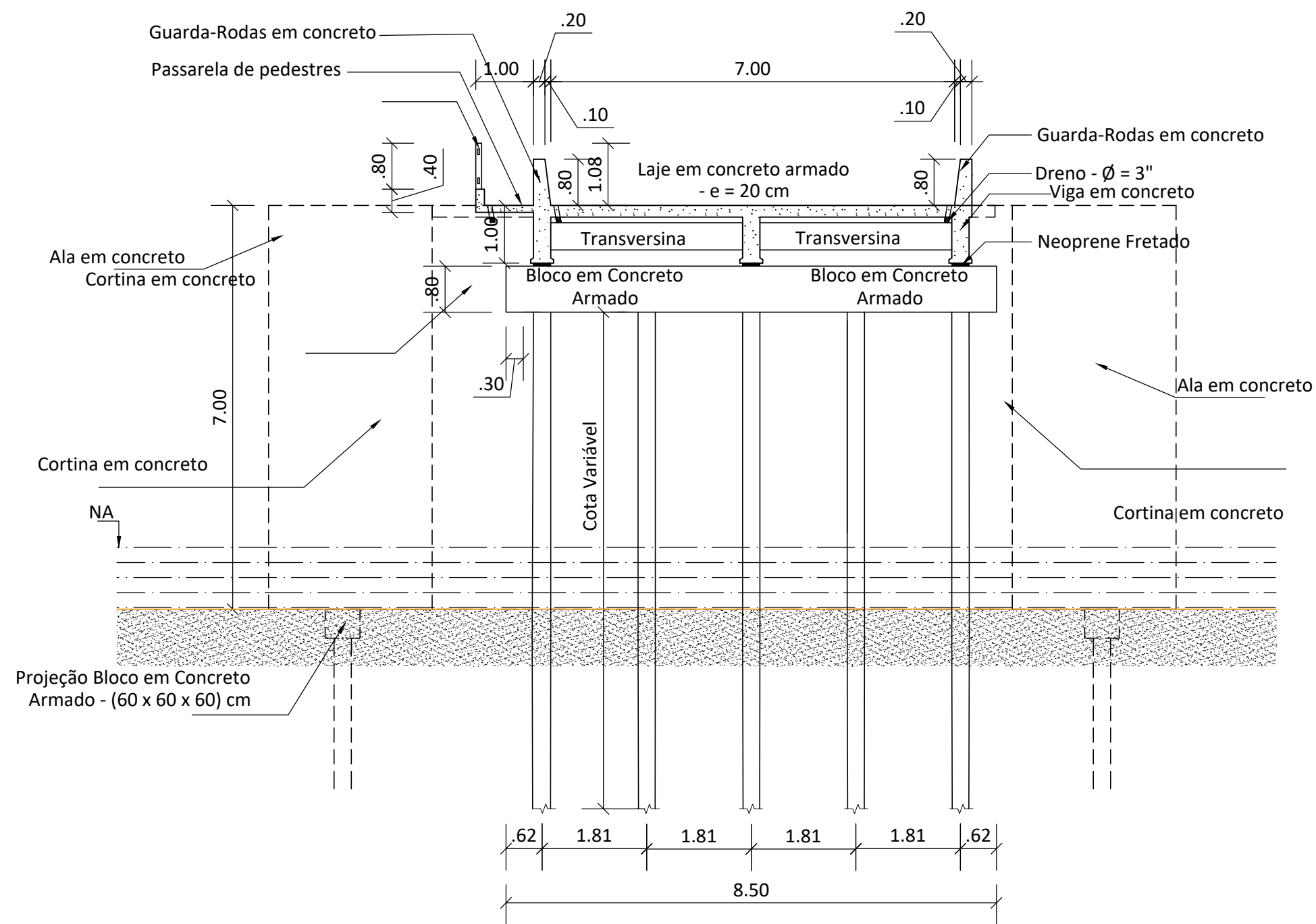
SEÇÃO 02 - TRANSVERSAL
