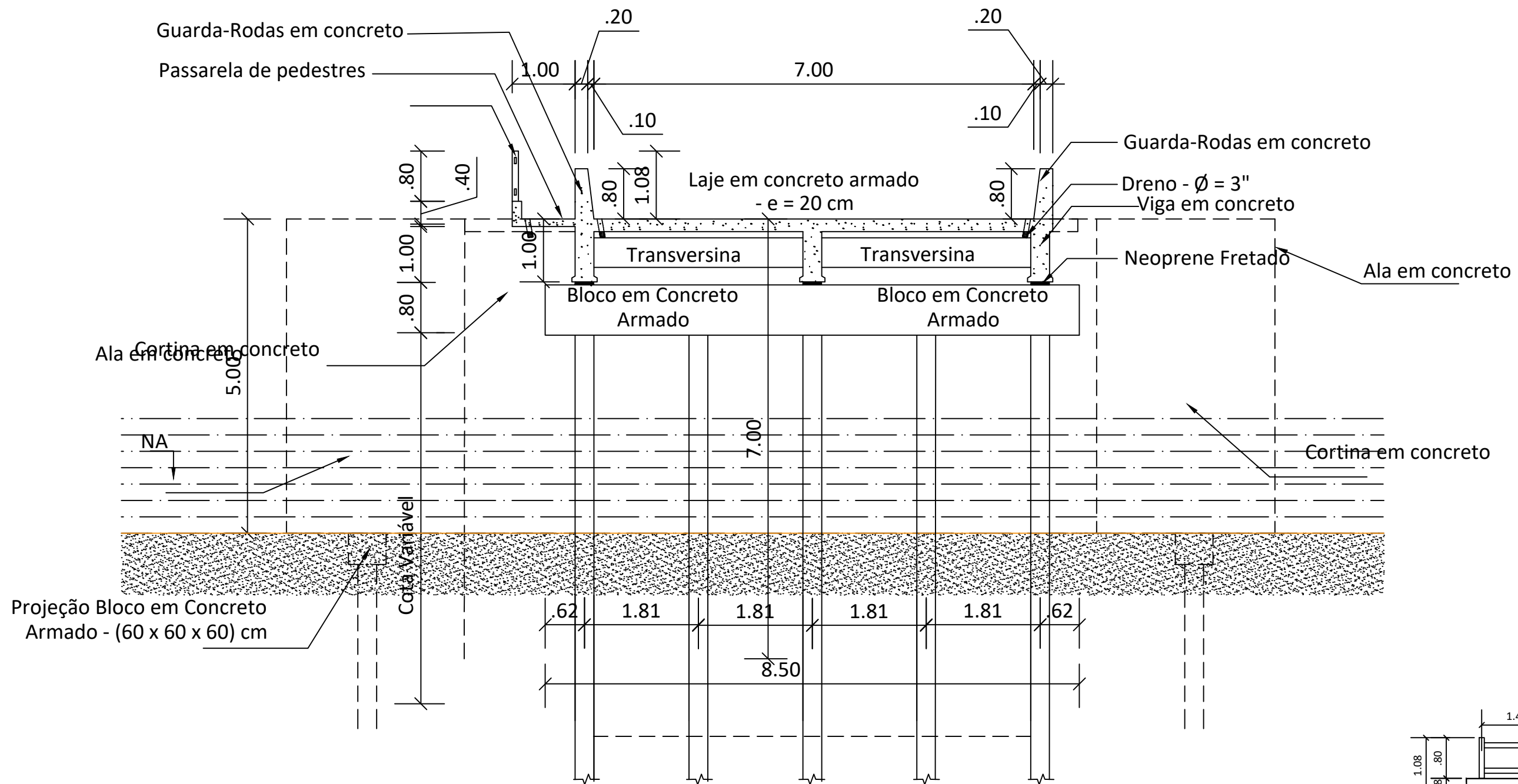
SEÇÃO 02 - TRANSVERSAL
