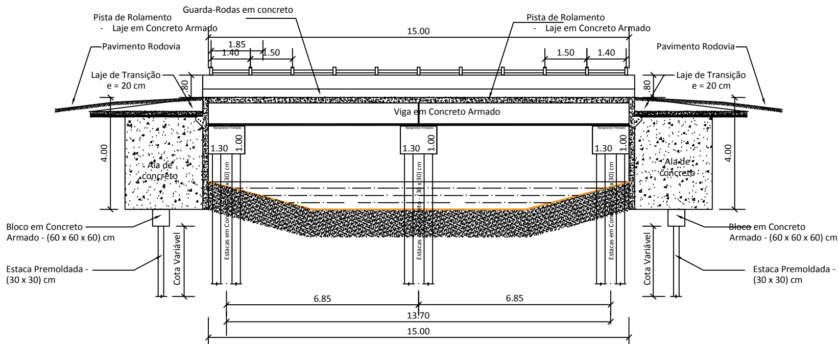
SEÇÃO 01 - LONGITUDINAL - ESCALA: 1 / 125
