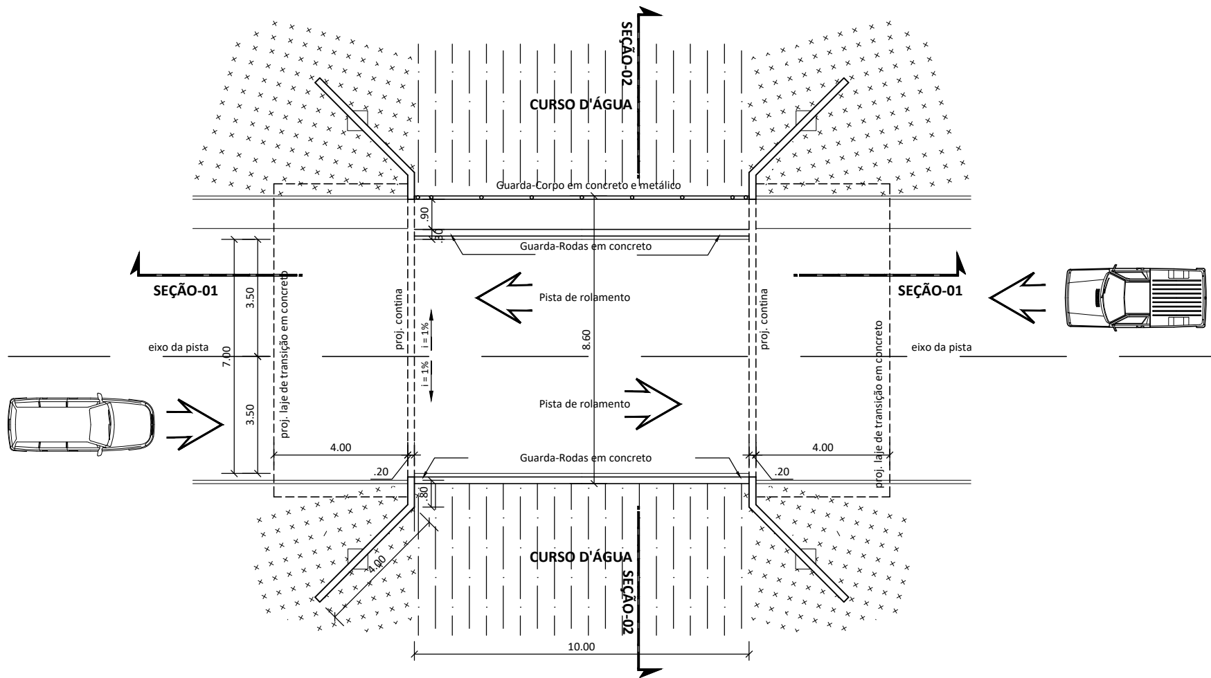
PLANTA ESQUEMÁTICA DA PONTE
