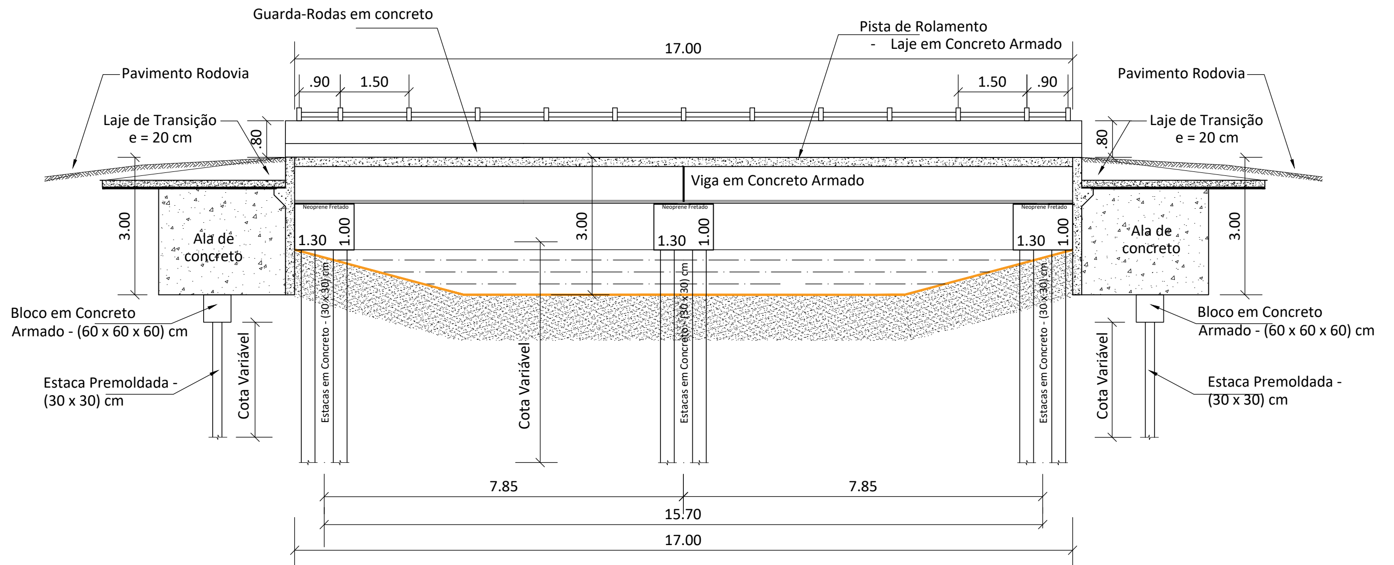
SEÇÃO 01 - LONGITUDINAL
