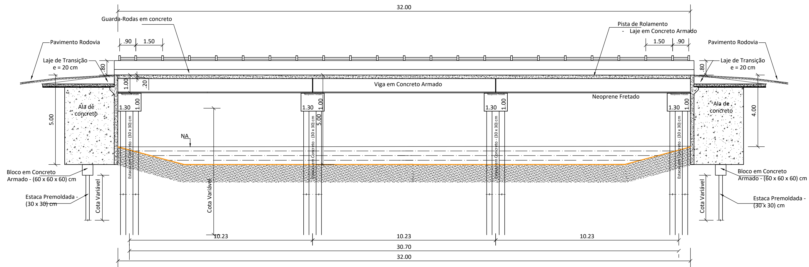
SEÇÃO 01 - LONGITUDINAL
