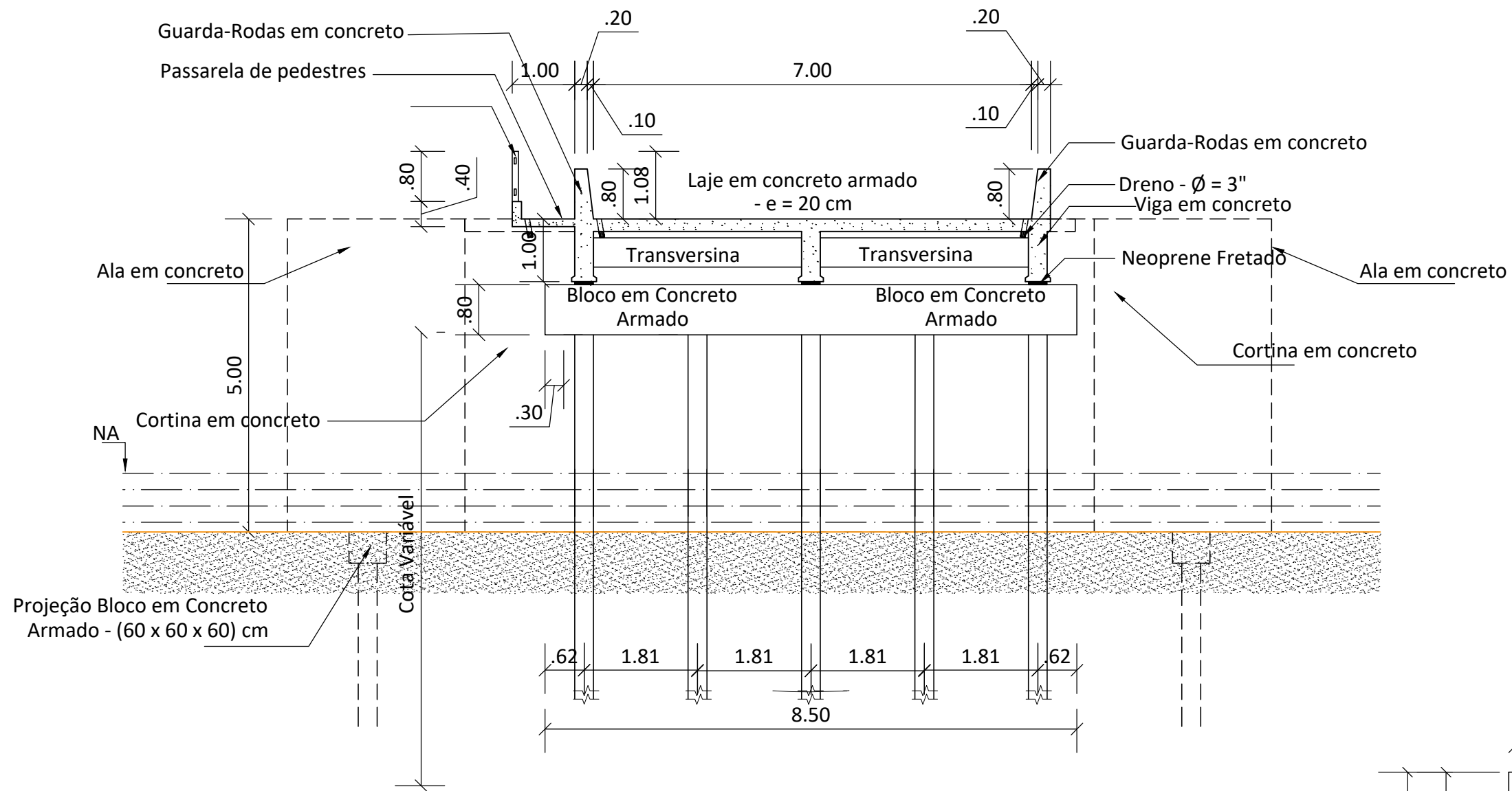
SEÇÃO 02 - TRANSVERSAL
