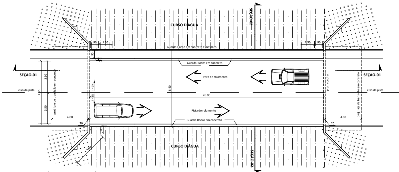
Planta Baixa esquemática
