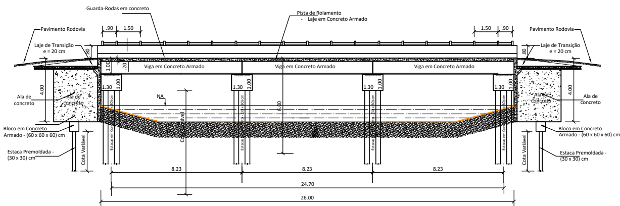
SEÇÃO 01 - LONGITUDINAL
