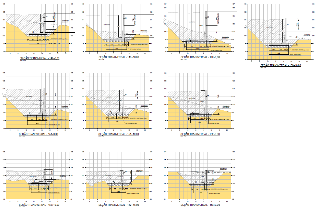
Figura 1 – Seções do Muro 2.
