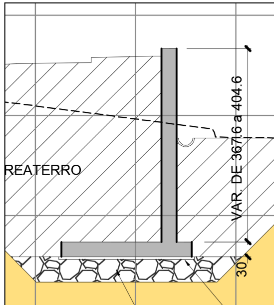
Figura 6 – Seção do muro de arrimo com destaque para as superfícies onde serão utilizadas formas.
