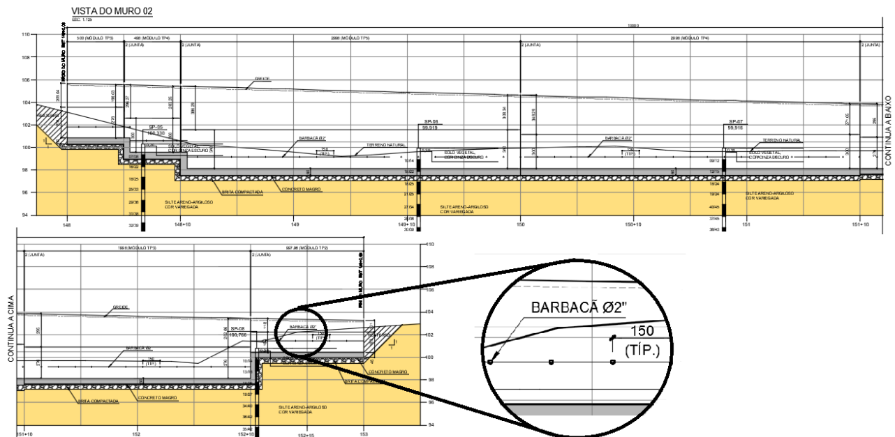
Figura 8 – Vista do Muro 2 com os barbacãs.
