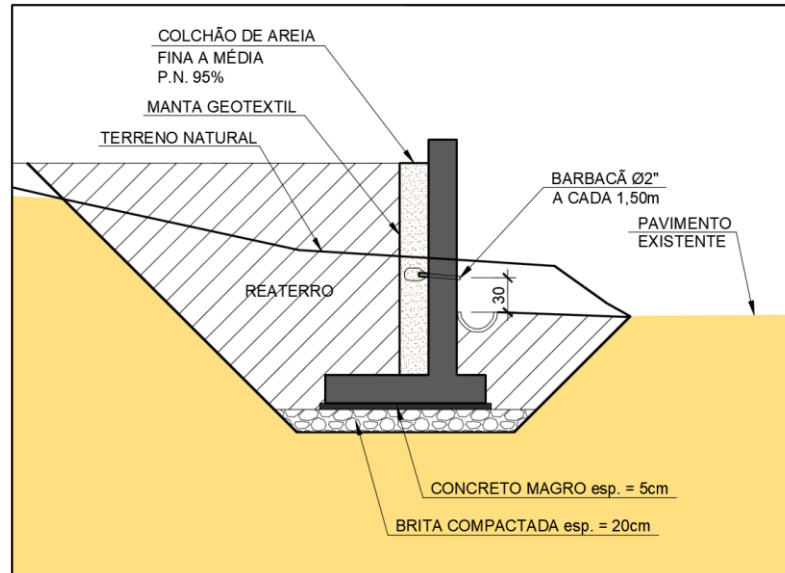
Figura 7 – Detalhe típico da drenagem do Muro 2.
