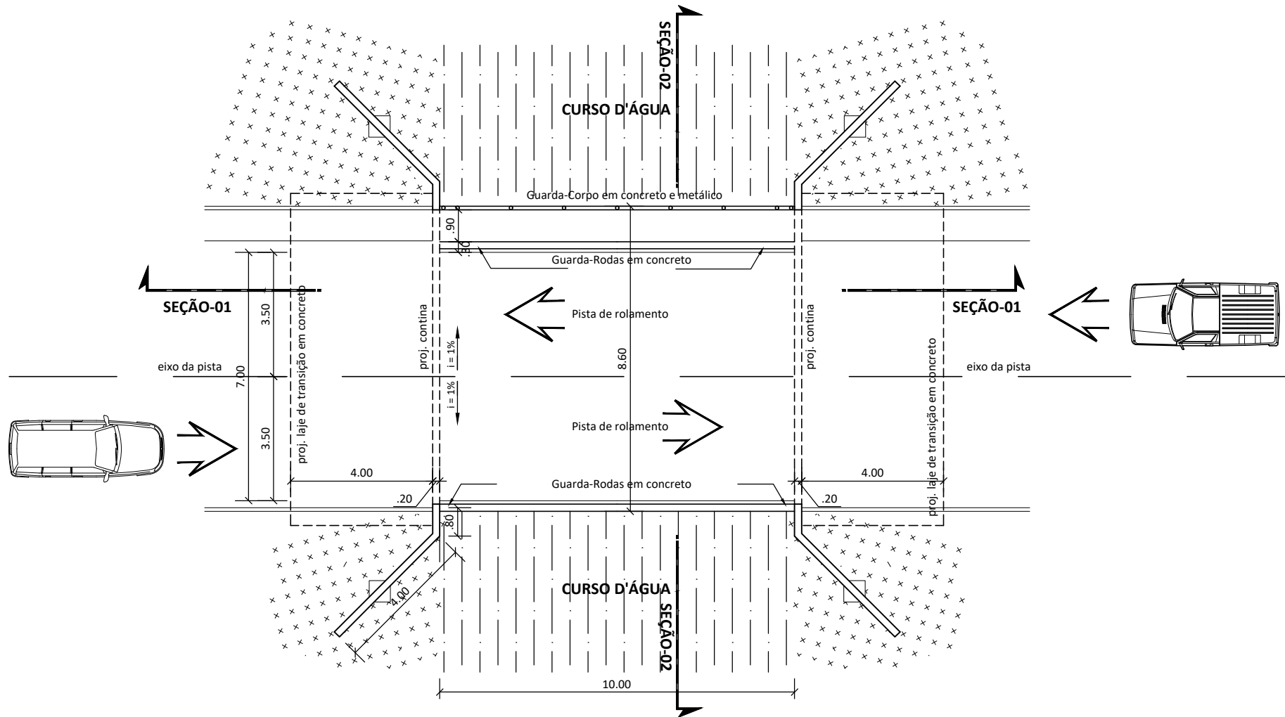
PLANTA ESQUEMÁTICA DA PONTE
