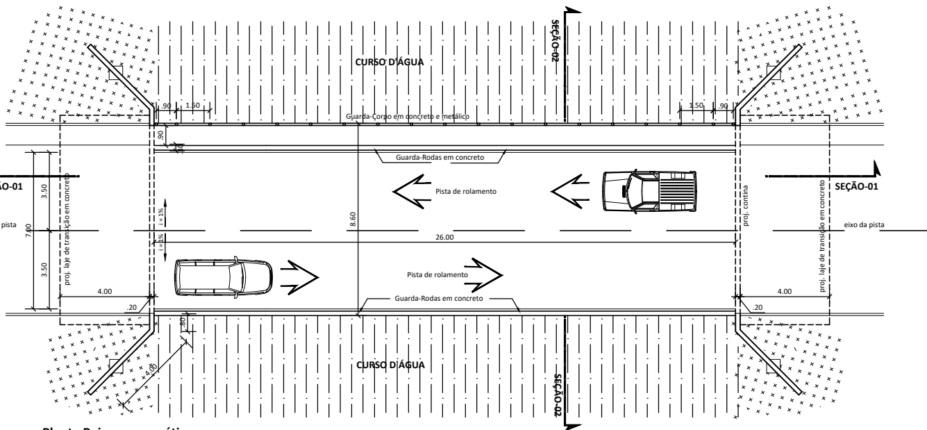
Planta Baixa esquemática
