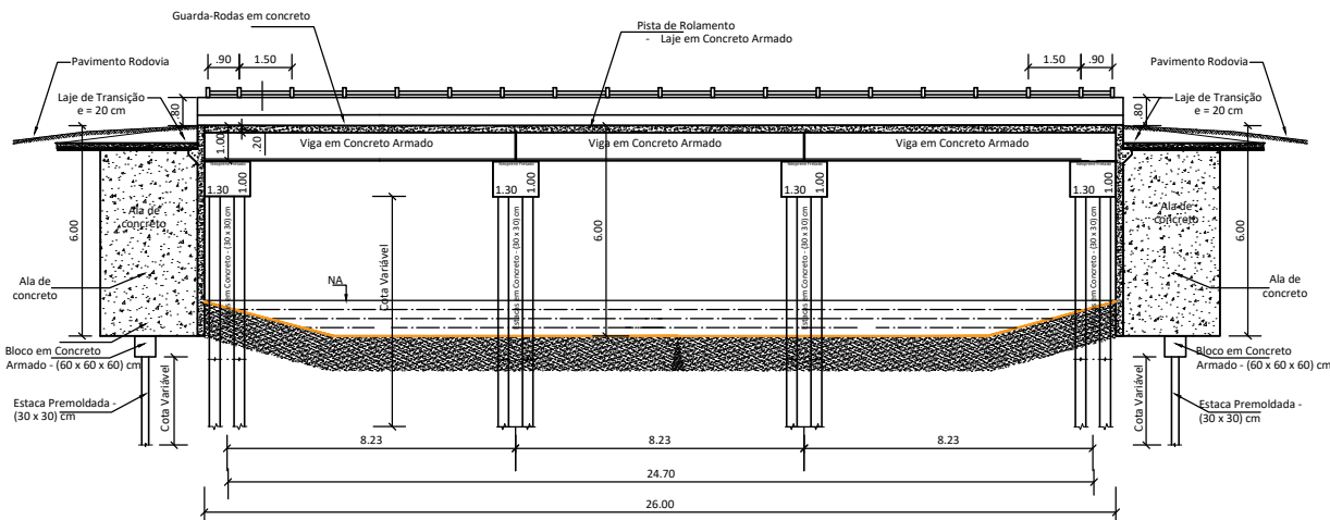
SEÇÃO 01 - LONGITUDINAL
