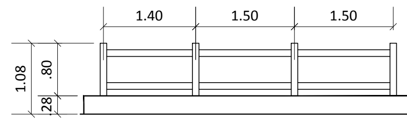
GUARDA - CORPO
