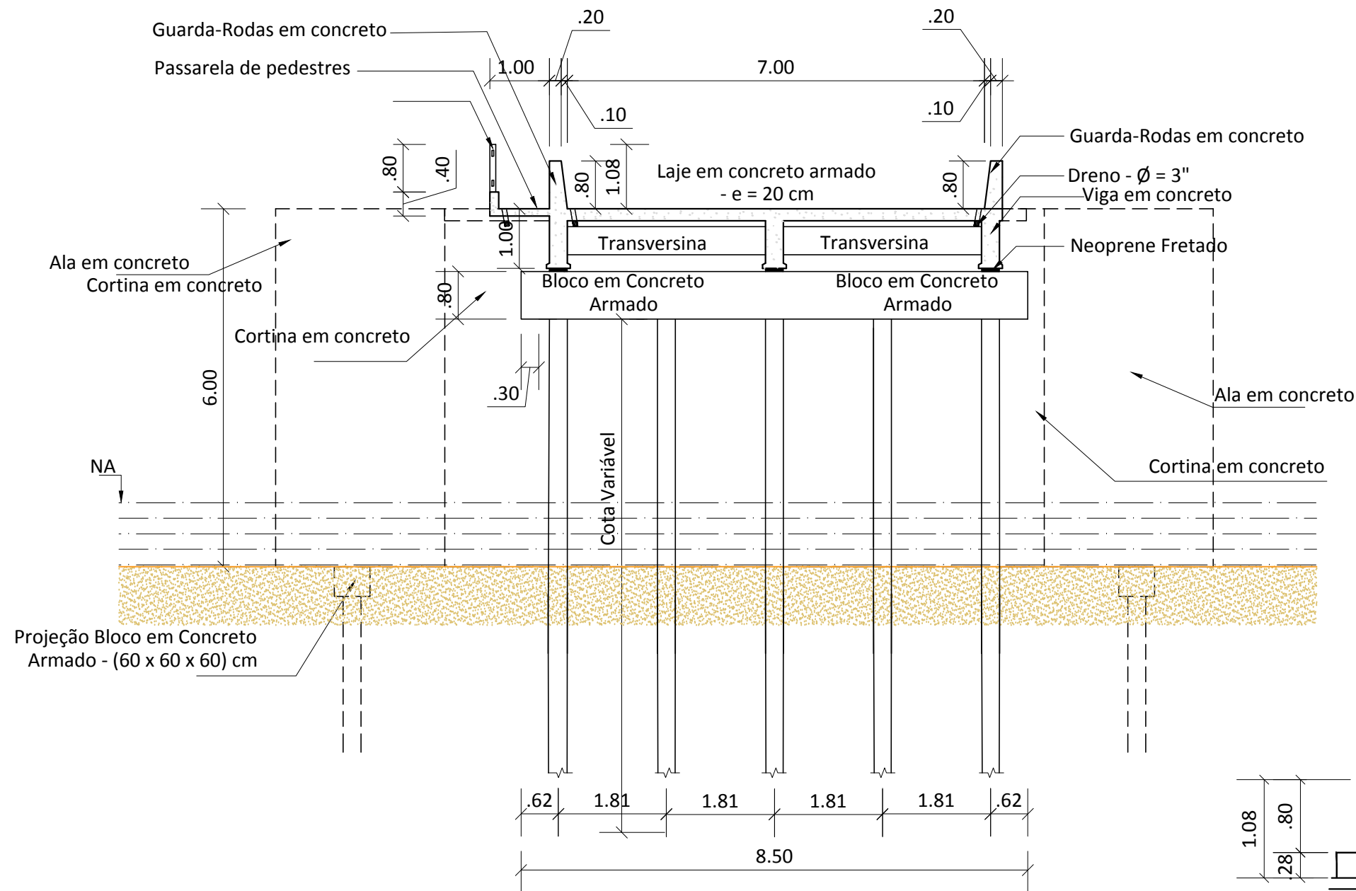
SEÇÃO 02 - TRANSVERSAL
