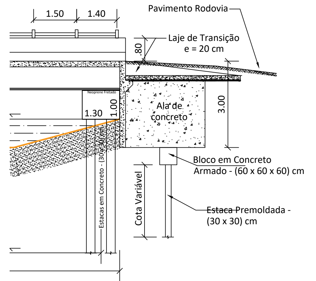
Pista de Rolamento - Laje em Concreto Armado
