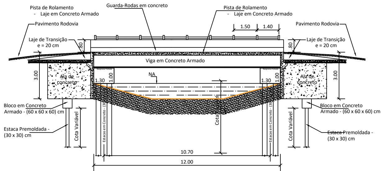
SEÇÃO 01 - LONGITUDINAL
