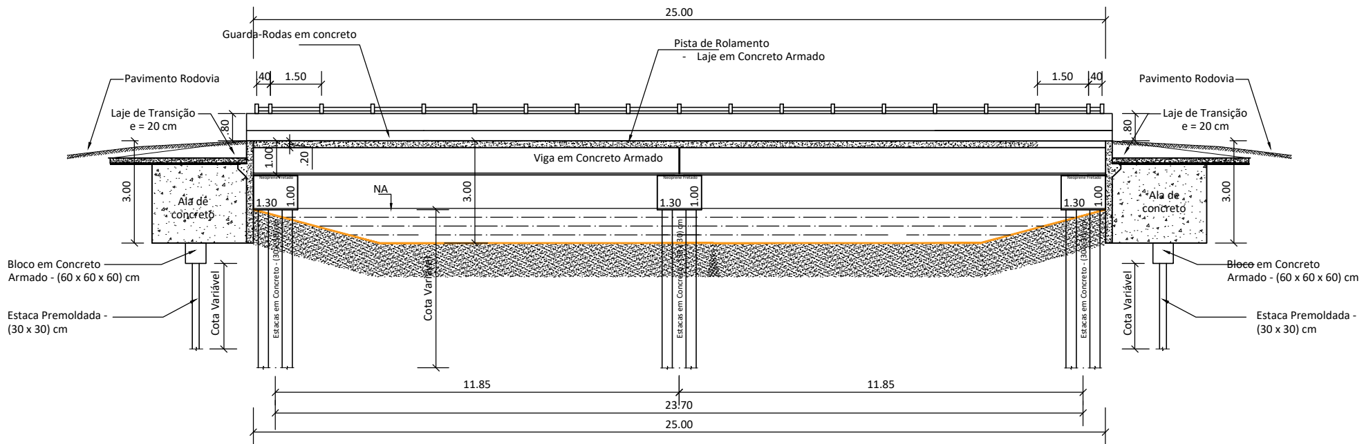
SEÇÃO 01 - LONGITUDINAL
