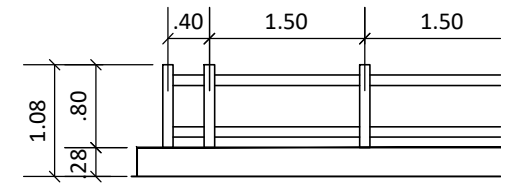
GUARDA - CORPO
