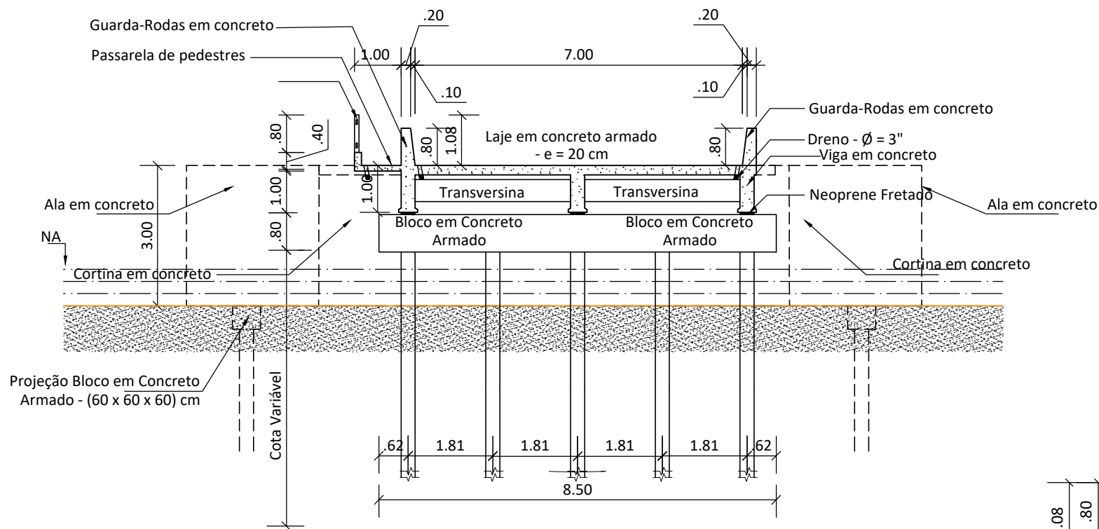
SEÇÃO 02 - TRANSVERSAL
