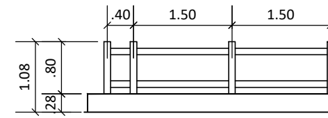
GUARDA - CORPO
