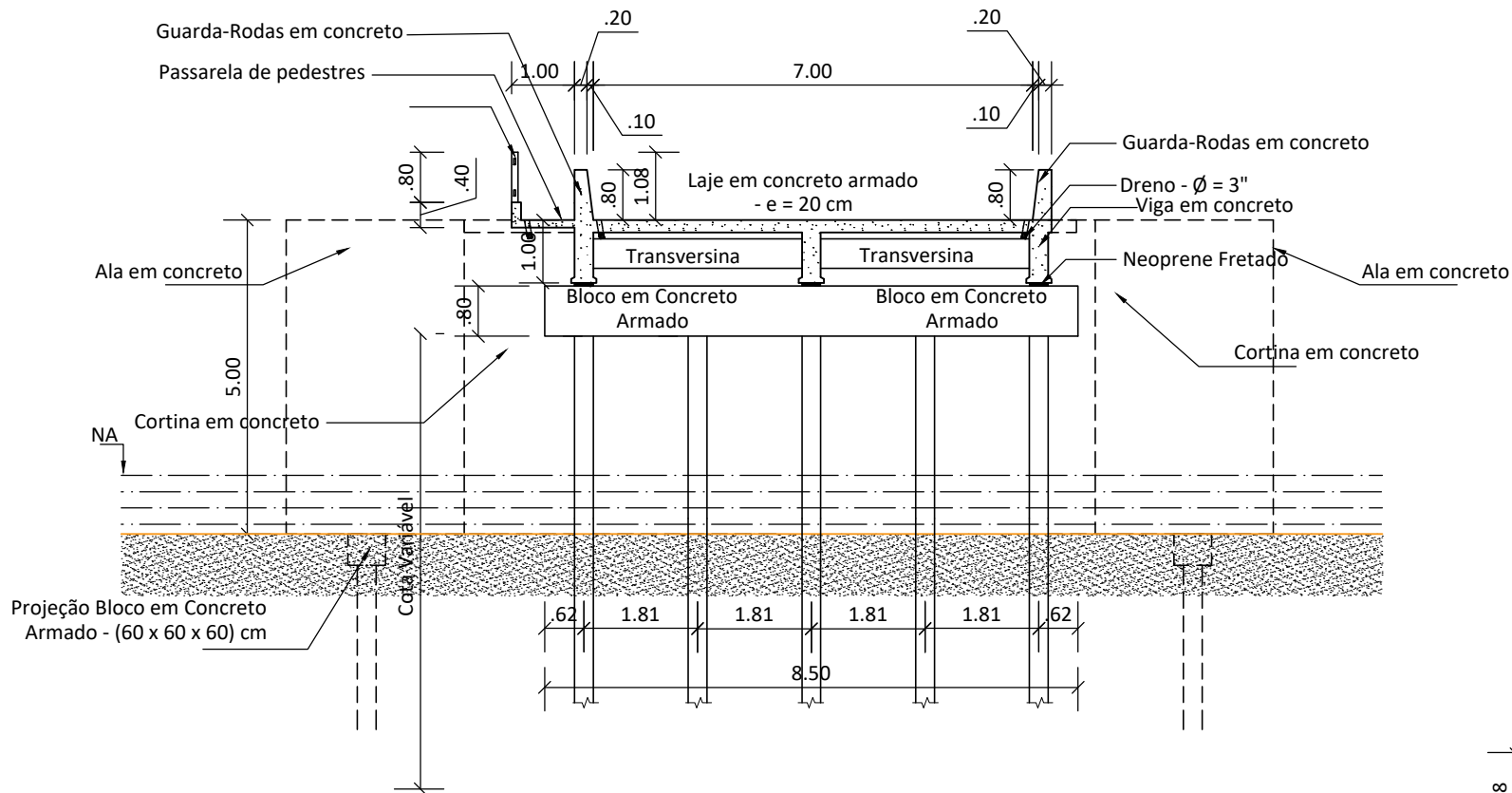
SEÇÃO 02 - TRANSVERSAL
