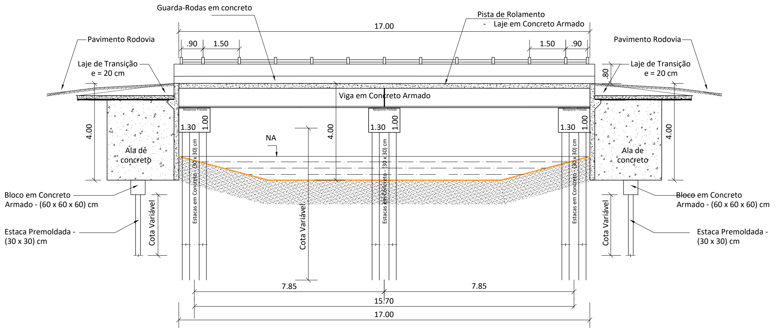
SEÇÃO 01 - LONGITUDINAL
