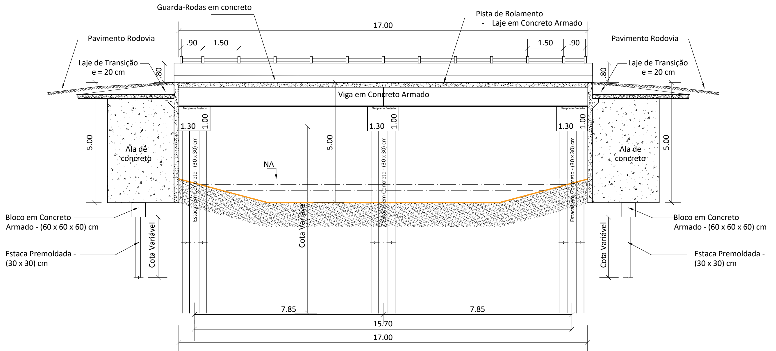
SEÇÃO 01 - LONGITUDINAL
