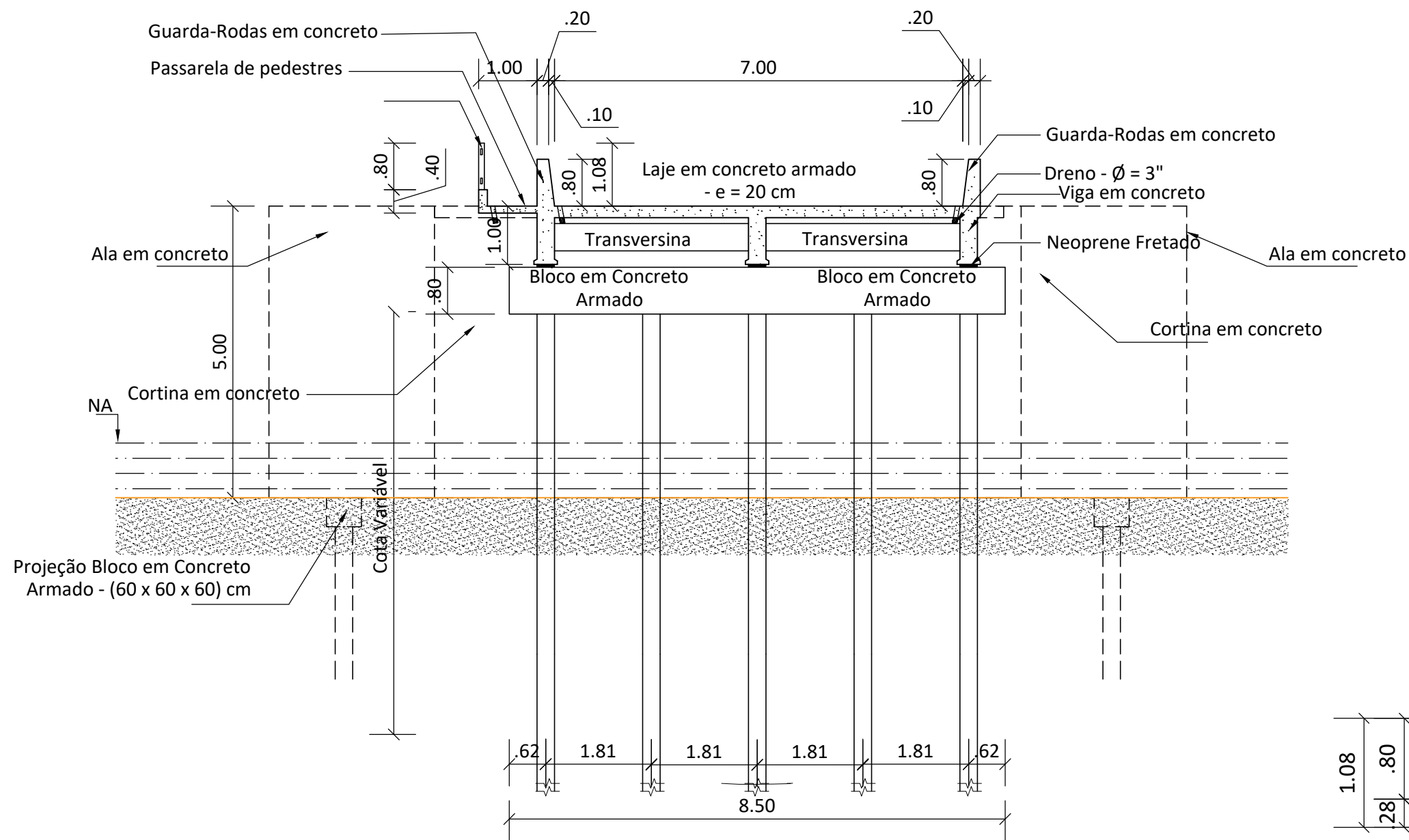
SEÇÃO 02 - TRANSVERSAL
