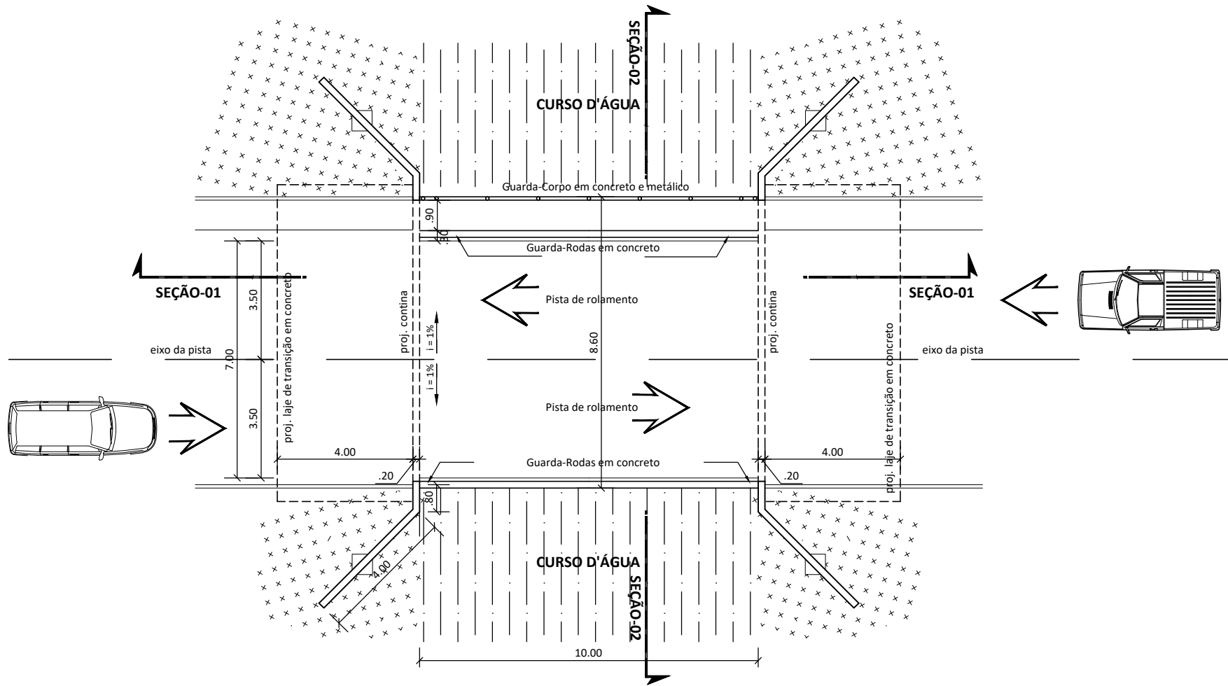
PLANTA ESQUEMÁTICA DA PONTE
